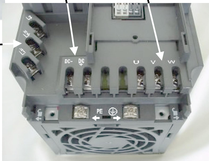
Obr. 7 Silové svorkovnice měničů velikosti B a C
