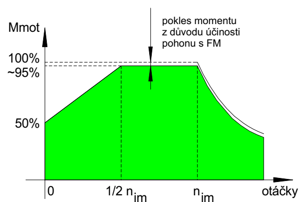
Obr. 14 Redukce zatěžovacího momentu motoru s vlastní ventilací
