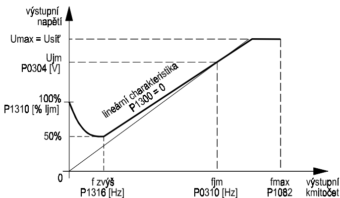
Obr. 42 Lineární charakteristika U/f
