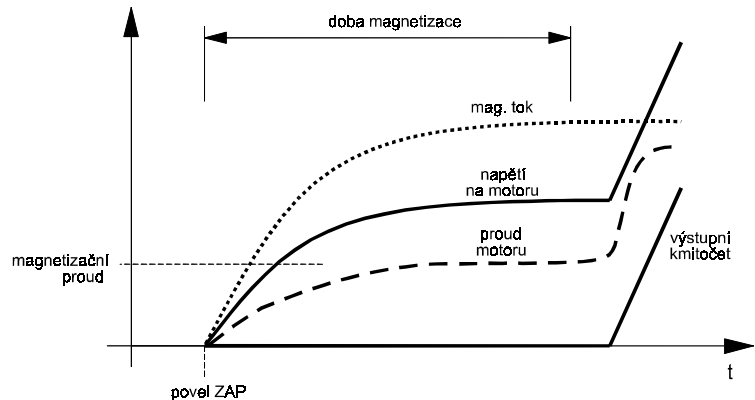
Obr. 49 Pozvolný nárůst magnetizačního napětí
