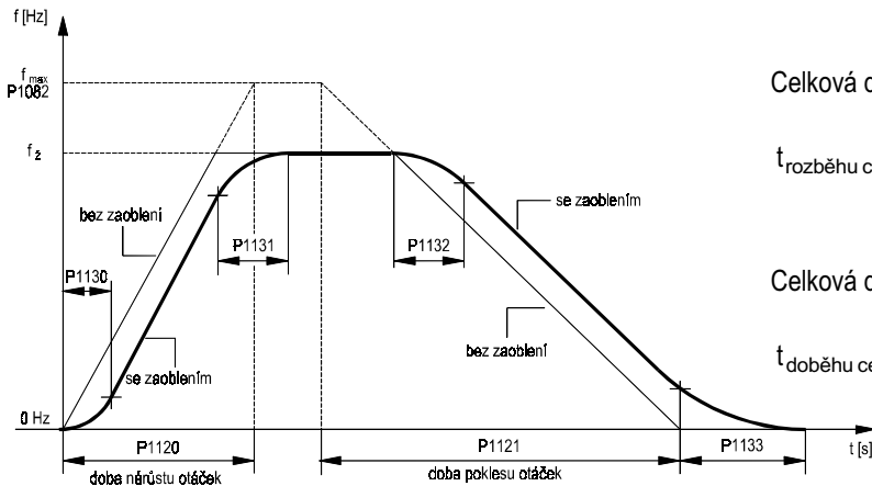
Obr. 37 Zaoblení křivky otáček
