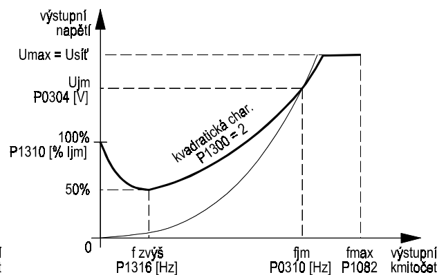
Obr. 43 Kvadratická charakteristika U/f
