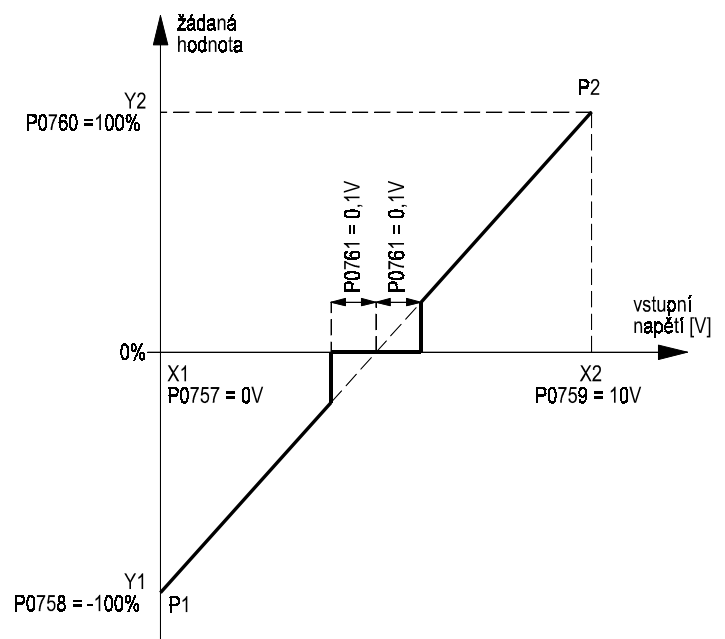
Obr. 28 Nastavení AIN pro zadávání směru otáčení analogovým signálem
