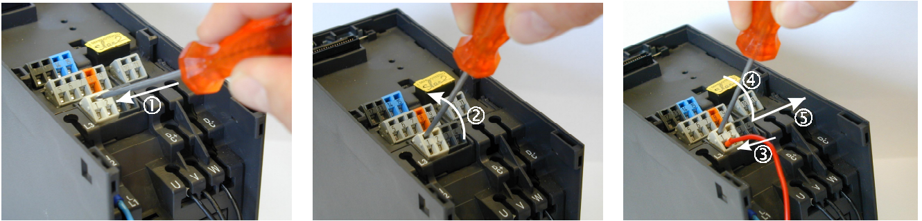
Obr. 13 Postup při upevnění vodiče v řídicí svorkovnici
