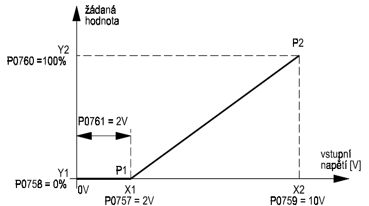
Obr. 27 Nastavení AIN pro proudovou smyčku 4 ÷ 20 mA
