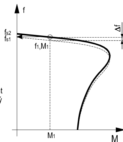
Obr. 47 Kompensace skluzu as. motoru
